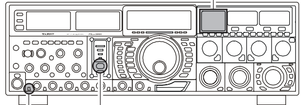
【R.FLT】 Switch 【ROOFING】 Switch
