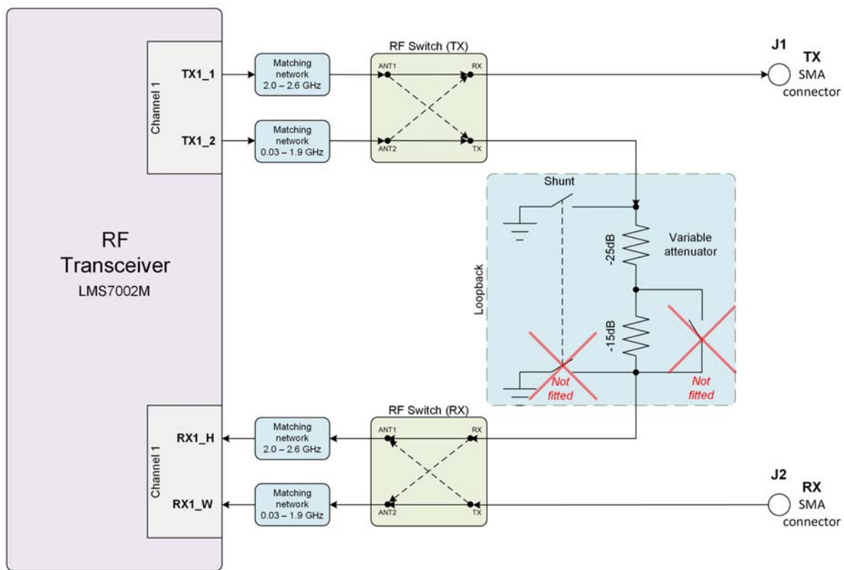
Figure 6: LimeSDR Mini v2.3 RF diagram
