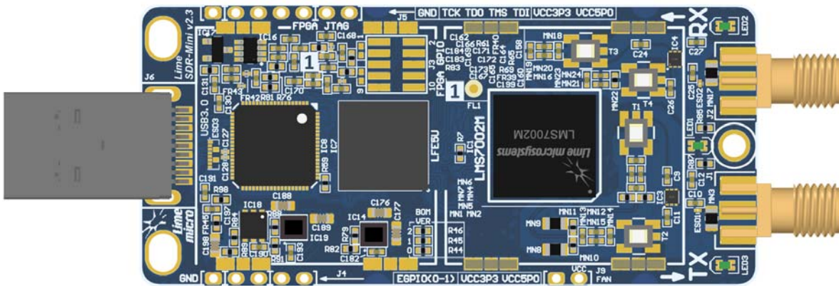
Figure 1: LimeSDR Mini v2.3 board top view
