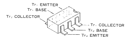
IMD2 (D2) (Q3009)
