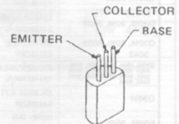
2SC2538 (Q4702)
