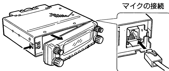
■コネクター接続部(正面から見た図)
