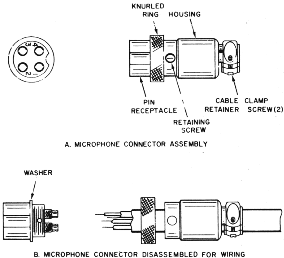
Fig. 2. Microphone plug wiring
