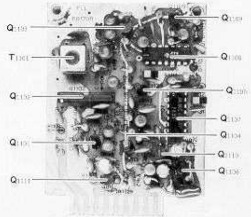
PLL unit (PB-1709A)
