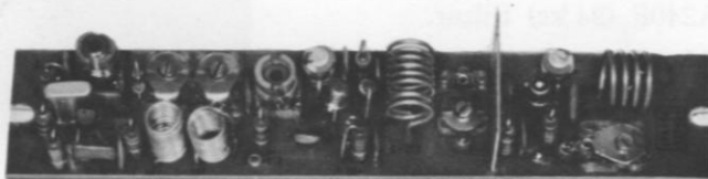
2 METER CONVERTOR
