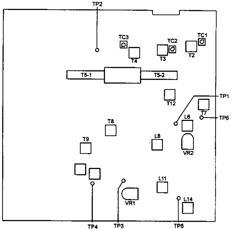
Linear PCB
