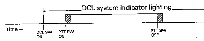
Fig. a. Simplex mode
