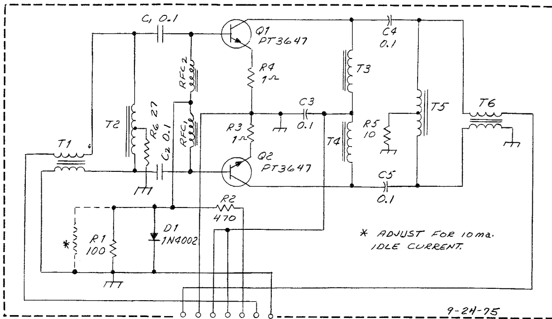
80185 R.F. POWER AMP.
