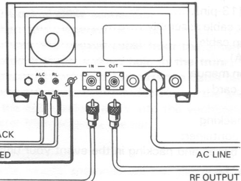
TL-922A
